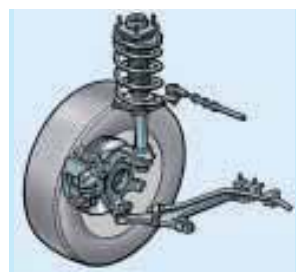
Train avant de type pseudo Mac Pherson : une précision optimale du guidage dans les courbes.
