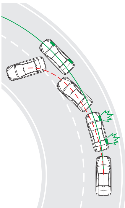
correction de survirage
